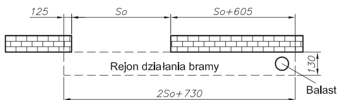
Wariant balastu B dla bram P-RB EI60
