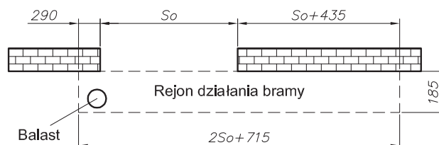
Wariant balastu A dla bram P-RB EI120
