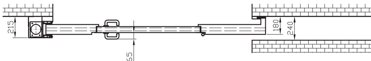
Dla bram P-RB EI120
