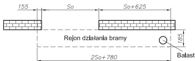
Wariant balastu B dla bram P-RB EI120
