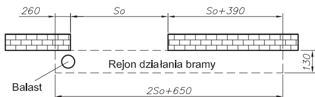
Wariant balastu A dla bram P-RB EI60
